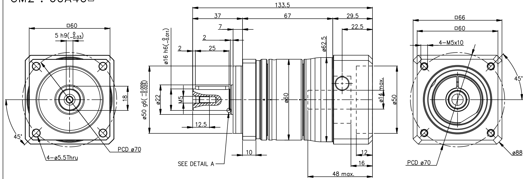
CM2 : 60A40□
