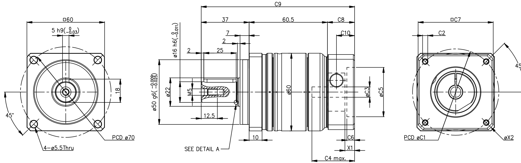
CM2 : 60A40□
