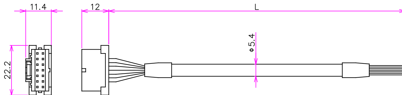
XADRP-14V (JST)
